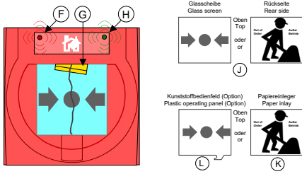
Abb. 4: Mechanische Alarmanzeige und LED, Glasscheibe, Papierinleger und Kunststoffbedienfeld Fig. 4: Mechanical alarm indicator and LED, Glass screen, paper inlay and plastic operating panel
